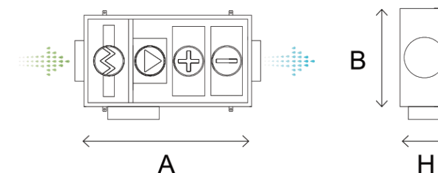
WIDOK Z GÓRY (przeciwny do strony obsługowej) WERSJA PRAWA TOP VIEW (opposite to the operating site) RIGHT VERSION
